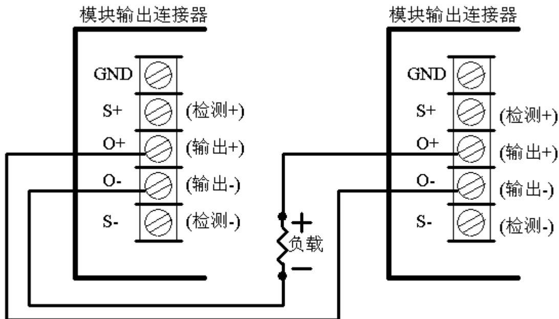
图 3-3 模块串联
