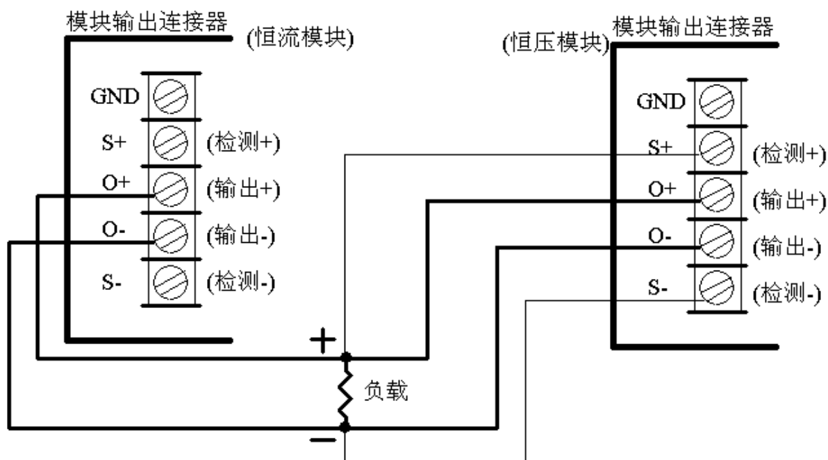
图 3-2 模块并联
