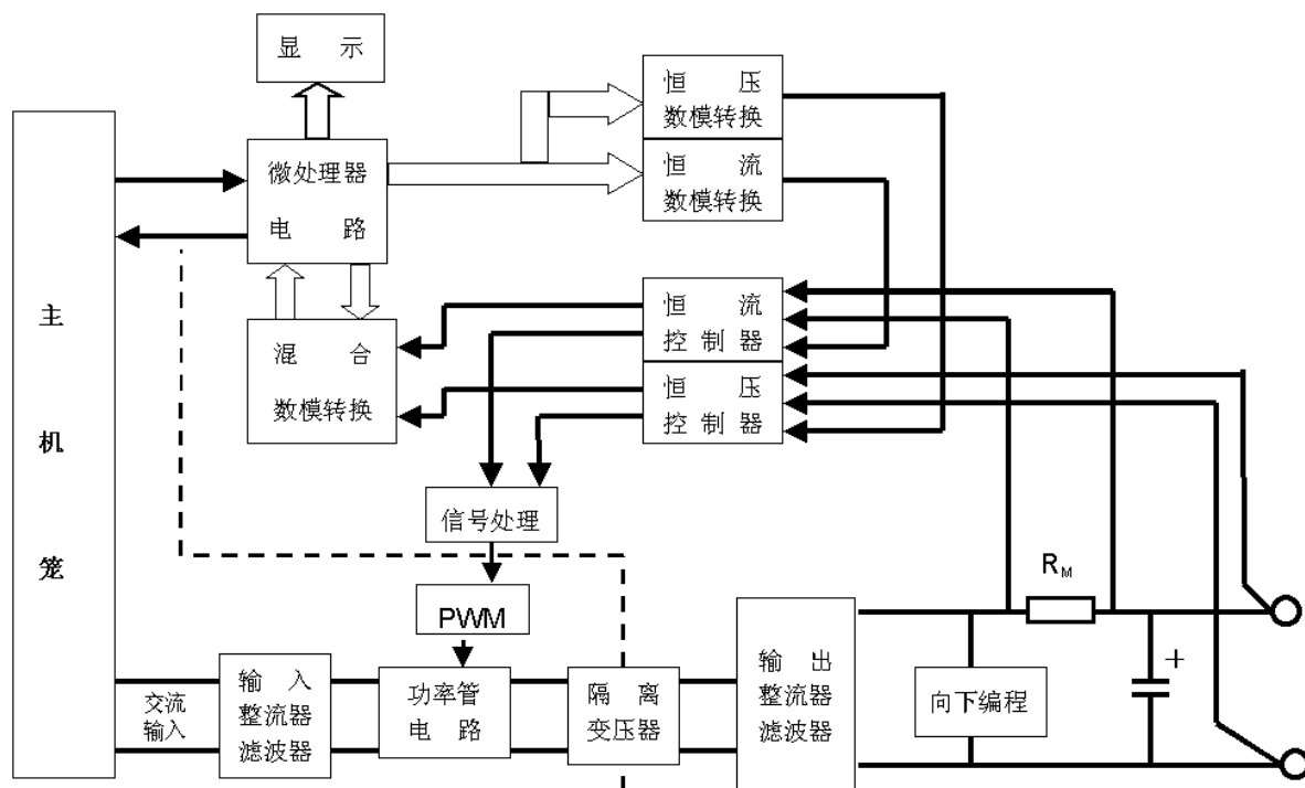
图 6-1 原理框图
