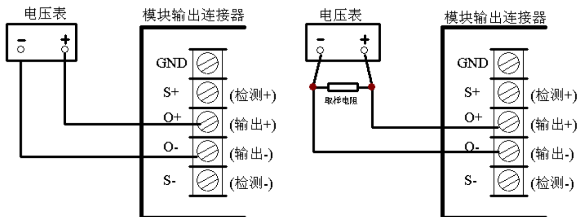
a) 电压校准
